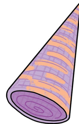
cone
