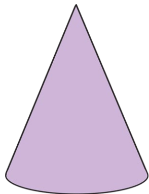
cone
