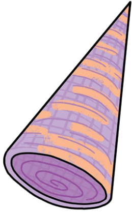
cone
