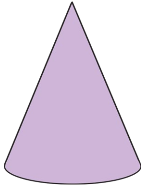
cone
