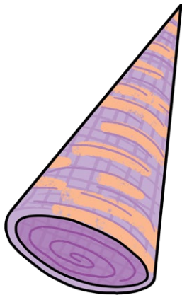
cone
