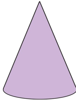
cone
